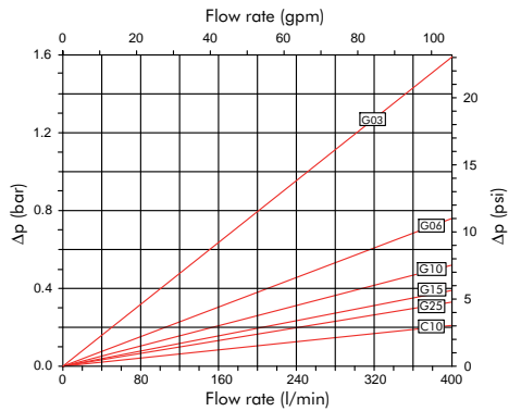
Element D143---A
